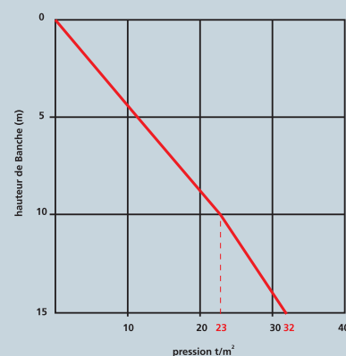
Pression sur les coffrages (coulage par le haut, cadence moyenne)
